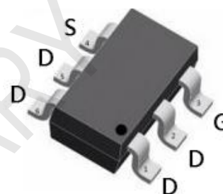
SOT-23-6
